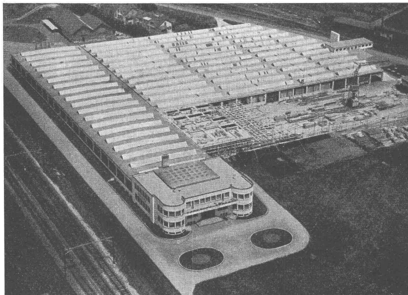
Traktoren- und Motorenwerke H. Hürlimann, Wil - Erweiterung 1946—1949, Flachbedachung 10 000 m 2 Bauleitung: F. Vogt, Architekt, Wil — Bauunternehmung: Ed. Züblin & Cie. A.-G., Zürich Eisenbetonarbeiten durch Fritz Meyer, Ingenieurbüro, Zürich 8
