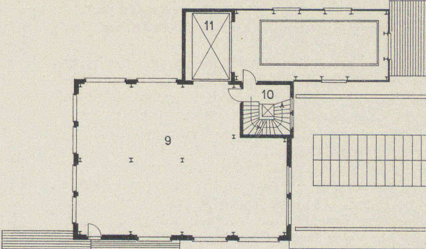
Bild 8. Zweiter Stock 1:400
