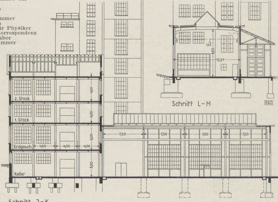
Schnitt J-K
