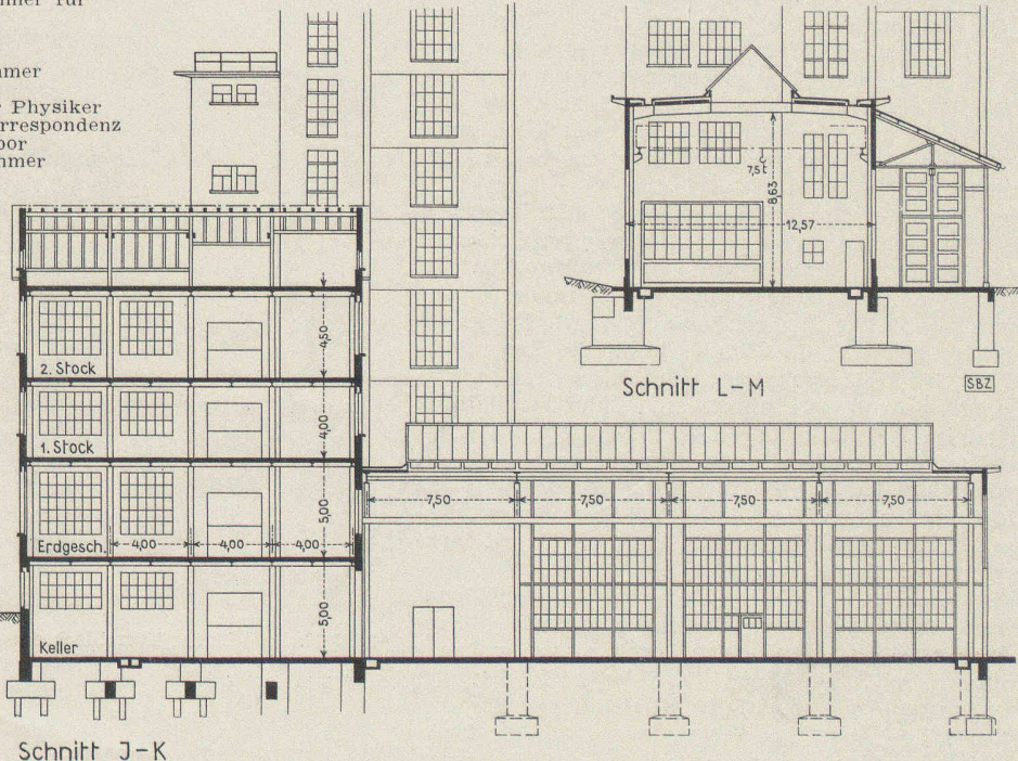
Schnitt J-K
