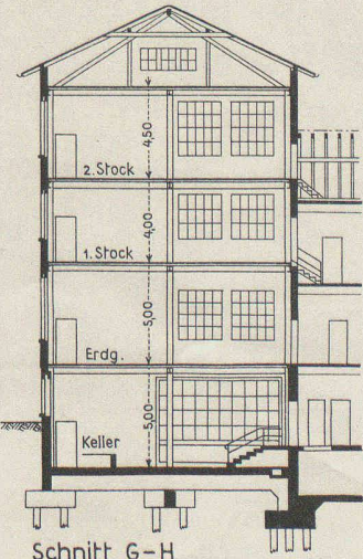
Bilder 9 bis 11. Schnitte 1:400
