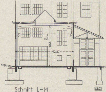
Schnitt L-M
