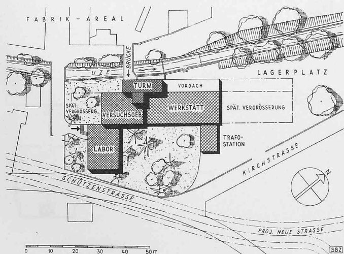
Bild 2. Lageplan 1:1500
