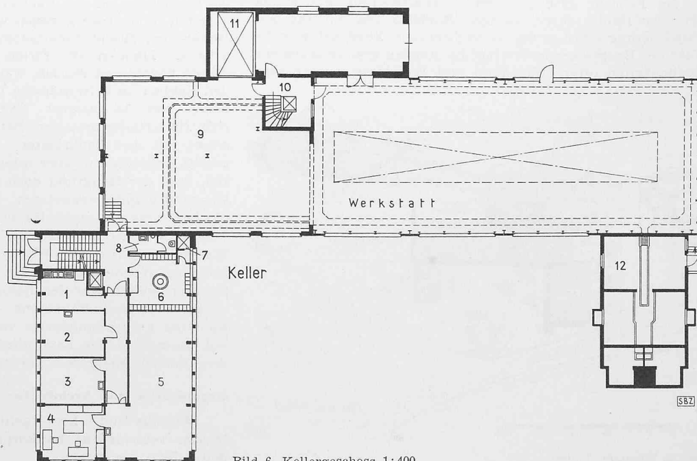
Bild 6. Kellergeschoß 1:400
