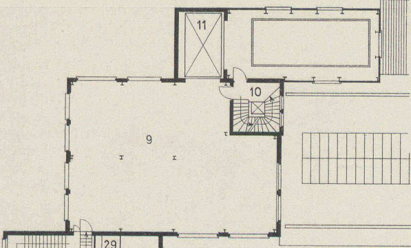
Bild 7. Erster Stock 1:400 (Müllerei-Labor)
