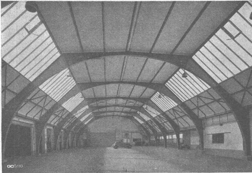
Auto - Einstellhalle
