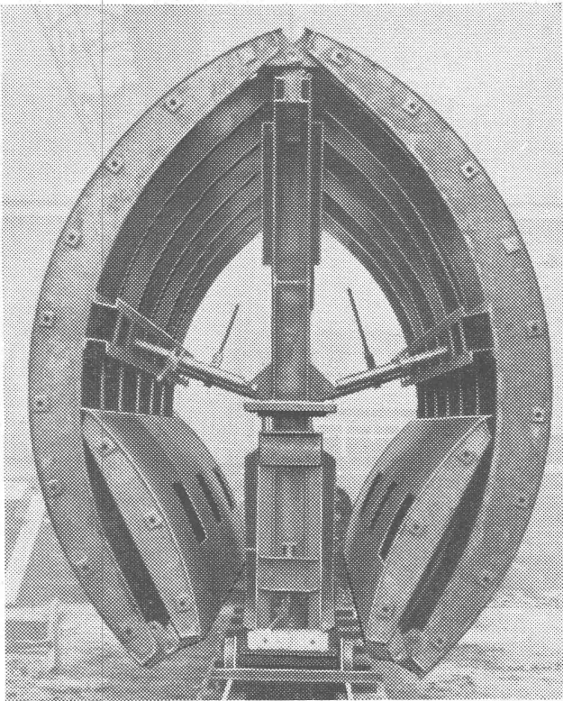
Teleskop-Stollenschalung \phi 3,75 m auf Transportwagen
