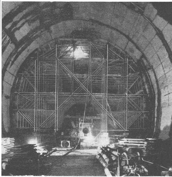
Fahrbares Lehrgerüst für Wasserschloss KW Lavey
