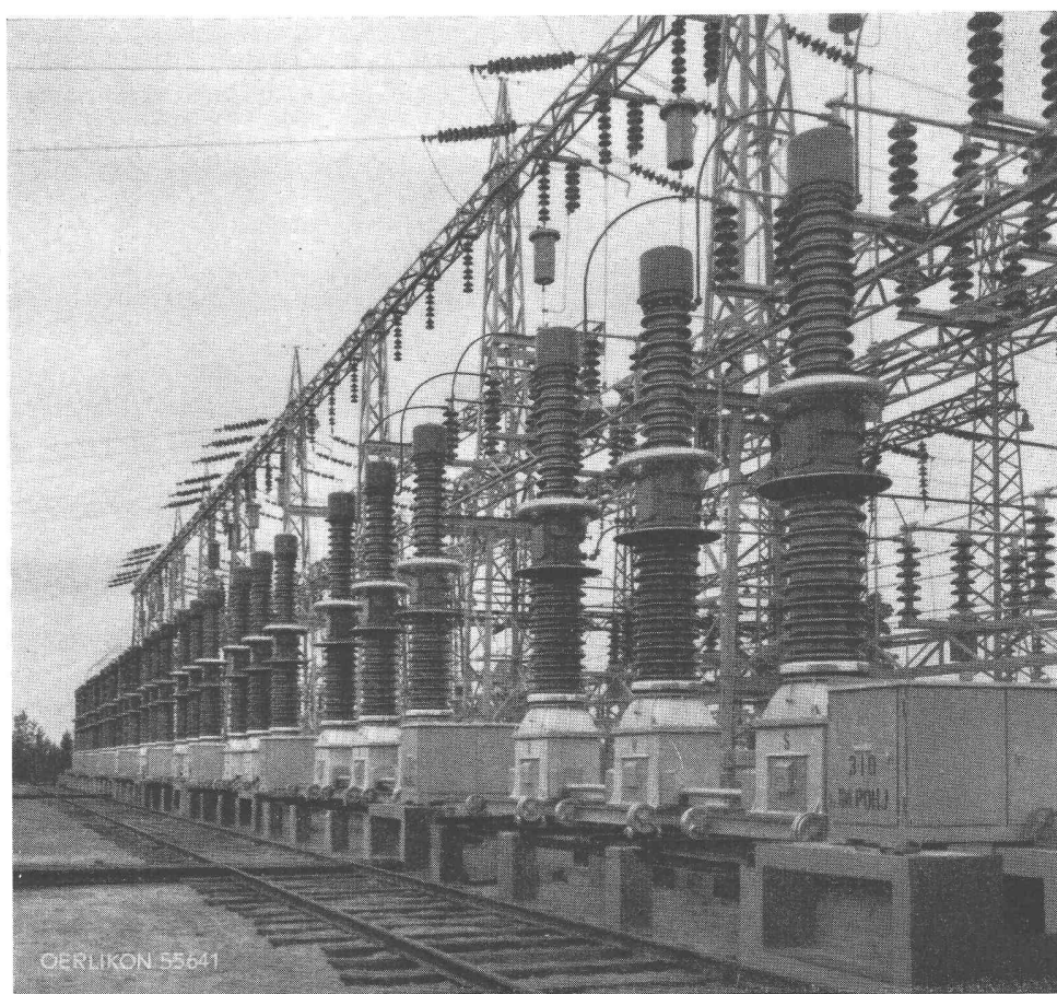
Gruppe von 9 ölarmen Schaltern, Typ TOF, 135 kV, 2500 MVA, in einer Transformatorenstation in Finnland.
