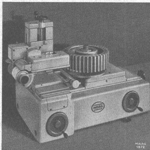
Zahnschrägemessgerät, Typ HM-30, für Stirn- und Schraubenräder bis 300 mm Durchmesser.
