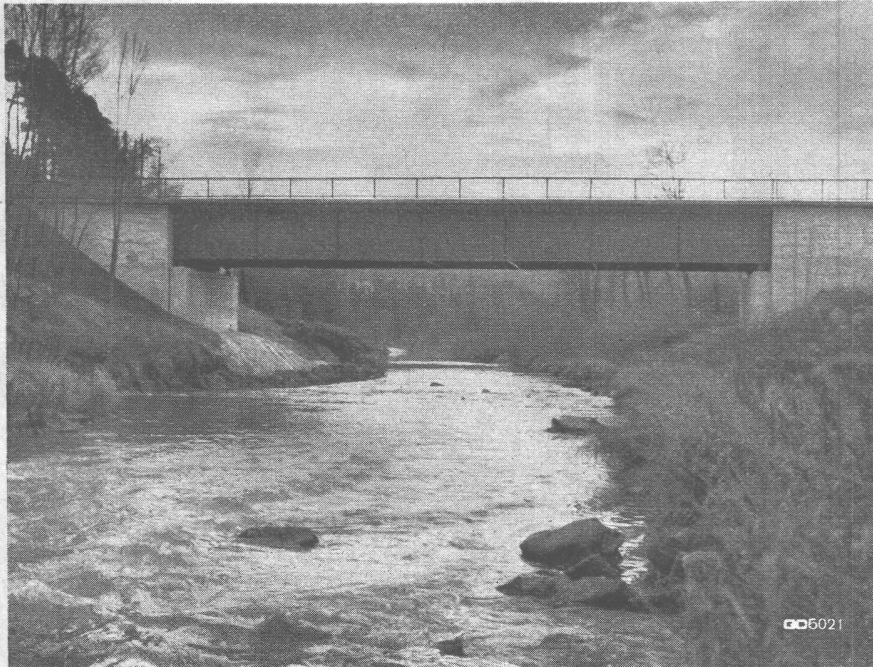
Tössbrücke Hard
