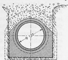
Schleuderbeton-Rohrleitung
