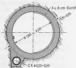
Bild 8. Querschnitte durch die Wasserführungsanlagen, Masstab 1:100
