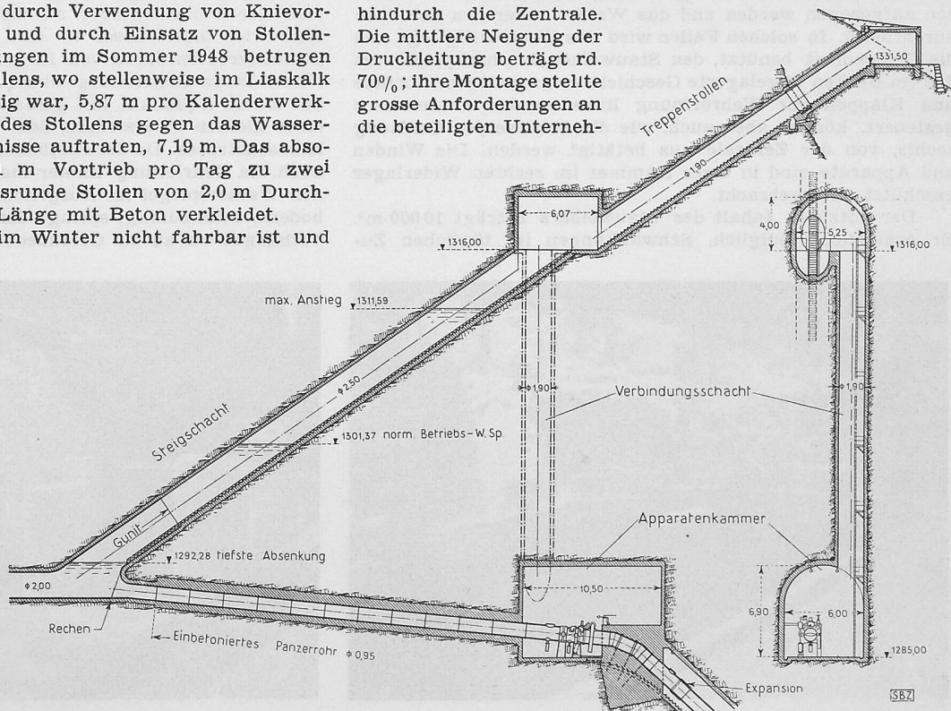
Bild 10. Wasserschloss mit Steigschacht und Apparatekammer, 1:500
