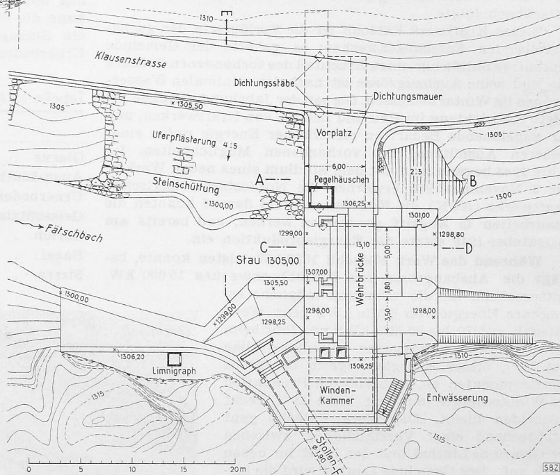
Bild 4. Stauwehr und Wasserfassung, 1:500
