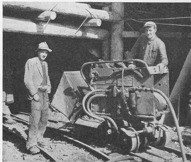
Bild 9. Stollenbagger
