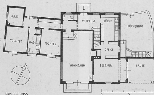
Bilder 3 bis 5. Grundrisse des Hauses im Grüt, Masstab 1:400
