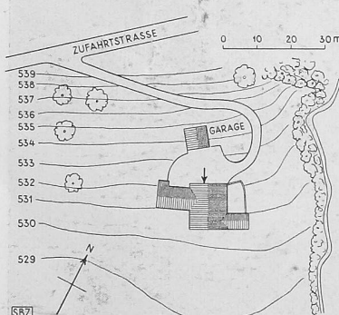
Bild 2. Lageplan 1:2000
