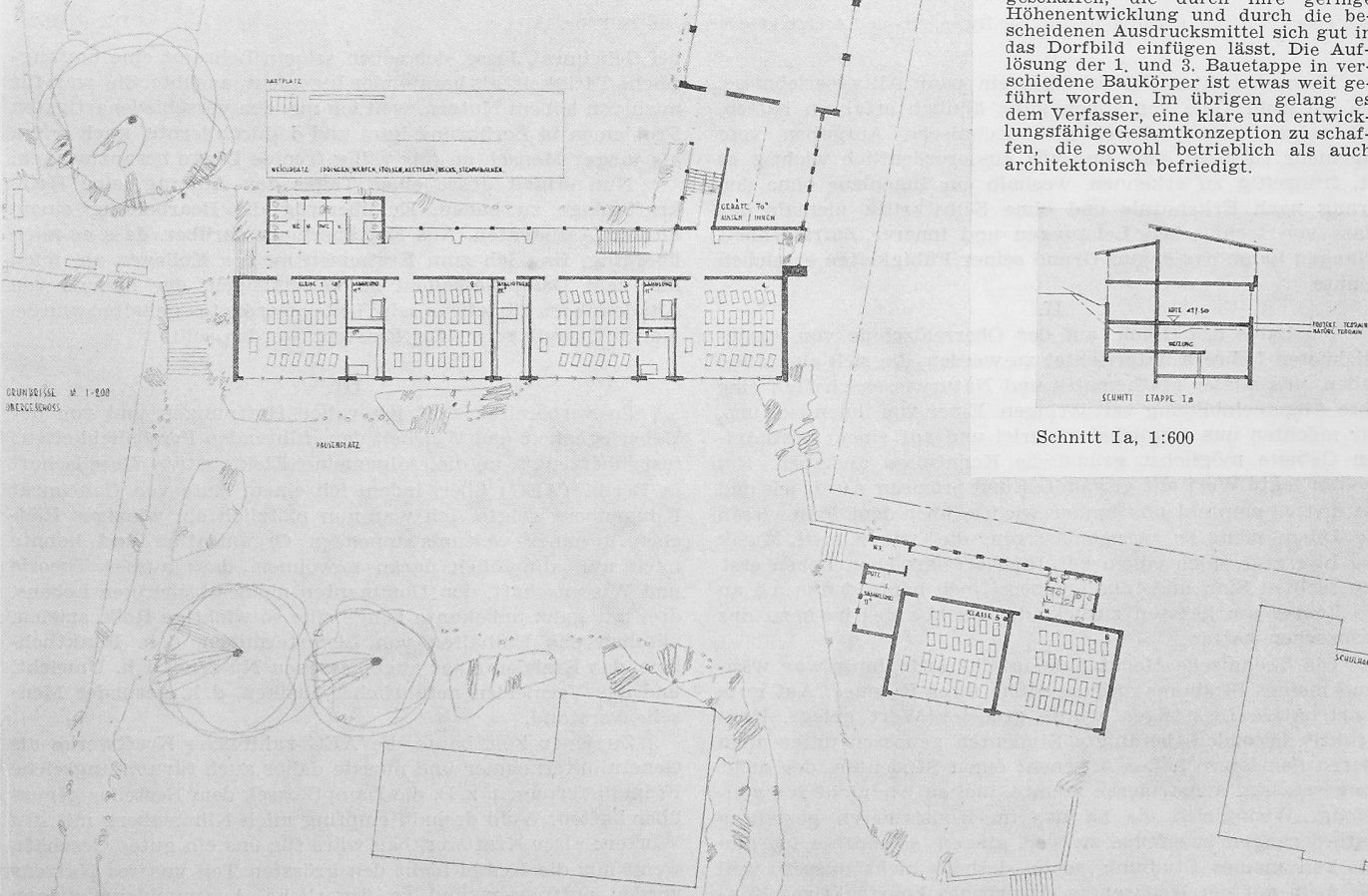
Obergeschoss Ia und Erdgeschoss Ib, 1:600. Ganz rechts das bestehende Schulhaus
