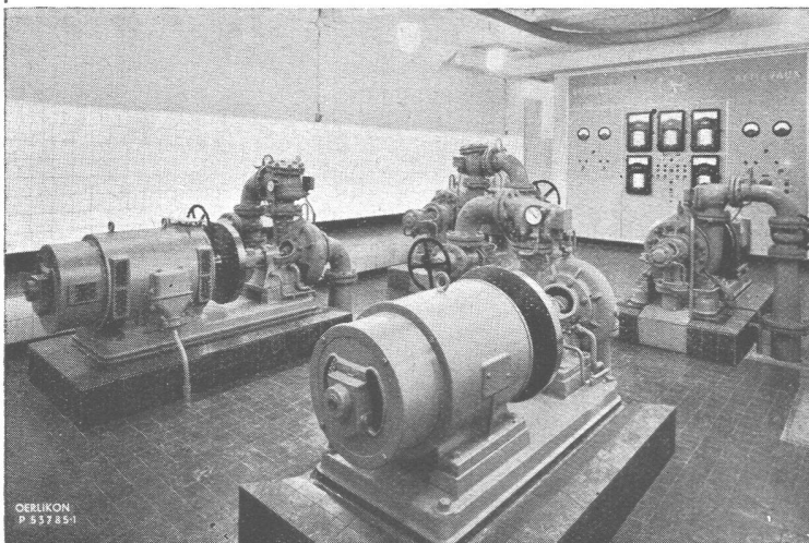
Trinkwasser-Pumpstation Calvaire bei Lausanne, ausgerüstet mit total drei Oerlikon-Combimotoren für 35, 55 und 75 PS.
