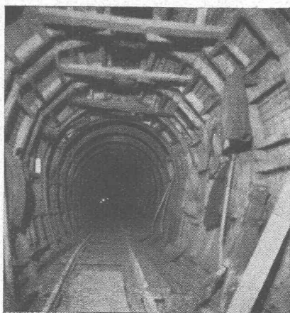
1140 m Stollen mit 30 lfm Schalung
