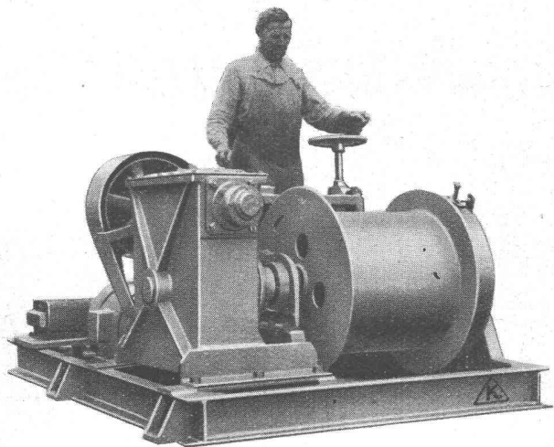
Type SG 60/50 mit Schneckengetriebe, mit kompletter elektrischer Ausrüstung
