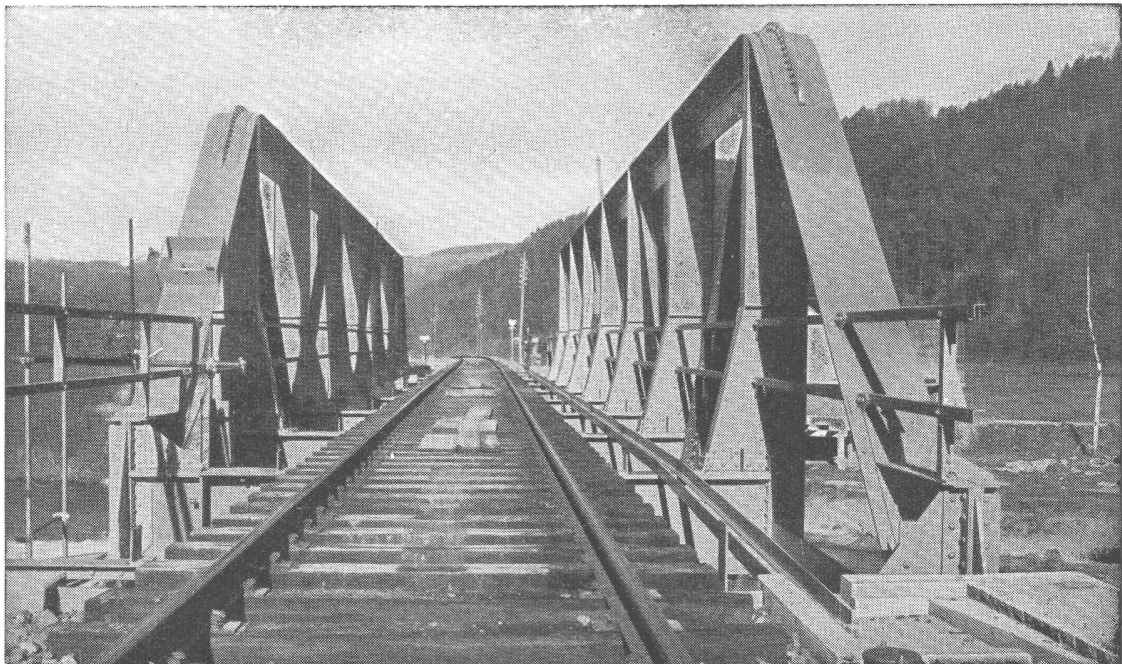
Tössbrücke Wila
