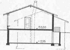
Bild 2. Schnitt 1:400
