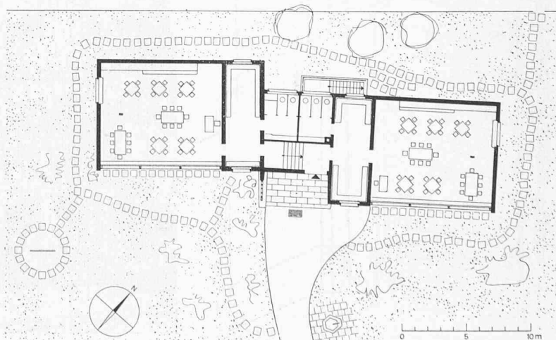
Bild 3. Grundriss 1:400
