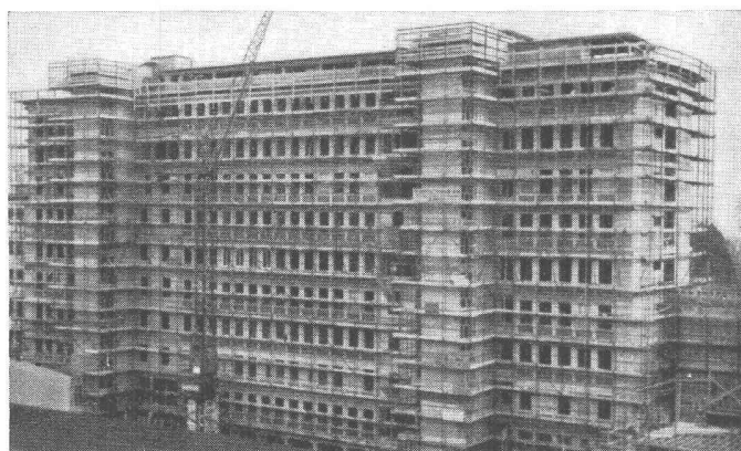
Bau- und Putzgerüst auf Konsolen, 35 m hoch
