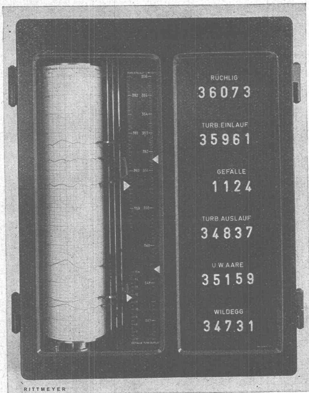
Kraftwerk Ruppertswil-Auenstein Registrierende Wasserstandsfernmelder für 5 Wasserstände und das Nettogefälle
