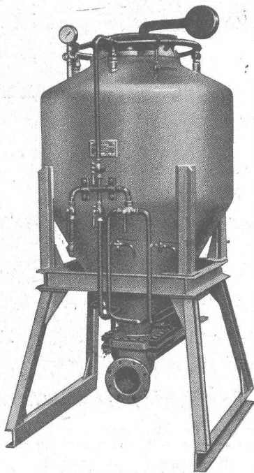
Betonier-Pneumatic zur hydraulischen Betonförderung
