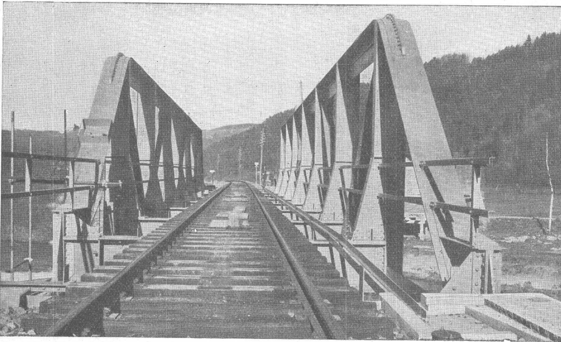
Tössbrücke Wila
