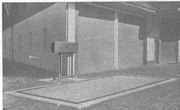
Brückenwaage für Strassenfahrzeuge, Wiegefähigkeit 15 t. Mit Betonbrücke, torsionsfreiem Hebelwerk und verstellbaren Schneiden
