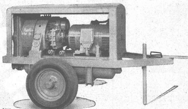
3016 Zweiradaggregat mit Luftkühlung und Elektromotorantrieb, 4,6 m 3 /min. eff.
