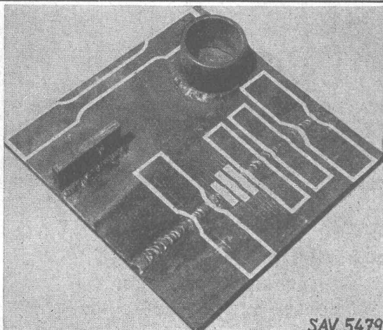
12 mm-Probplatte für die Schweisserprüfung nach VSM 14061
