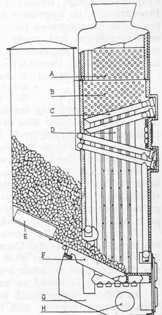
Dampferzeuger u. Kohlenbunker A Rauchgasvorwärmer, B Ueberhitzer, C Quersiederöhre, D Verdampferrohre, E Kohlschieber, F Rost, G Aschkasten, H Öffnung für Verbrennungsluft
