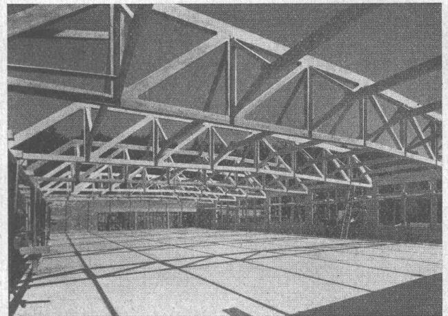
Eisenbetonfachwerk - Montagefertig
