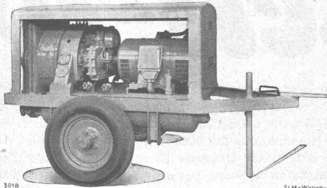
3018 Zweiradaggregat mit Luftkühlung und Elektromotorantrieb, 4,6 m 3 /min. eff. SLM-Winterthur
