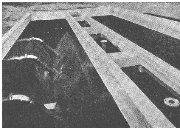
Kläranlage der Stadt Zürich. NEROL-Anstrich auf Zementglattrich.
