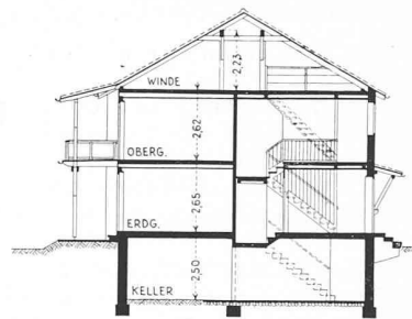
Bild 7. Grundrisse und Schnitt der Zweifamilienhäuser im «Schachen»; Masstab 1:300
