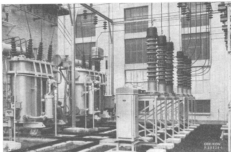
Freiluft-Transformatoren- und Schaltstation in der Zuckerfabrik Aarberg mit elektrischer Ausrüstung Oerlikon. — Links zwei Dreiphasen-Transformatoren von je 10 000 kVA, der eine für 50/6 kV, der andere für 50/16 kV mit Lastschalter. Rechts zwei dreipolige ölarme Schnellschalter für 50 kV Betriebsspannung. 600 A, 750 MVA.
