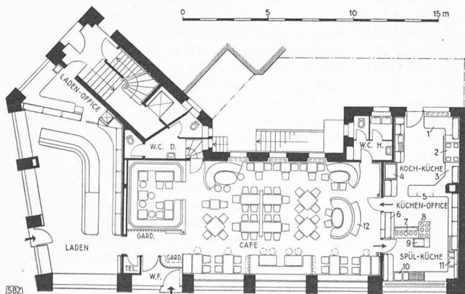
Bild 1. Grundriss 1:300. Legende: 1 Rüsten, 2 Kochen (bestehend Gasher), 3 Anrichten, 4 Kühlschrank, 5 Wärmeschrank, 6 Getränke, 7 Kaffeemaschine, 8 Glace, 9 Reg.-Kasse, 10 Gläser-spüle, 11 Geschirrspüle, 12 Besteck. — Laden siehe Seite 126
