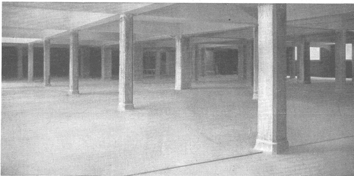
Ca. 600 m 2 wasserdichter Barra-Zementüberzug auf Kellerboden 6 m unter Strassen-Niveau
