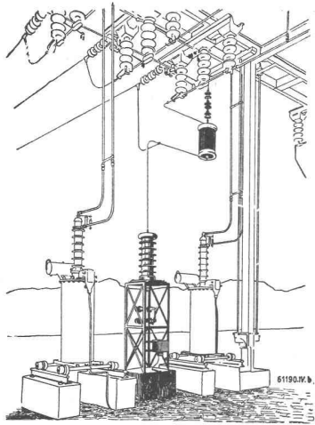
HF-Telephonieschrank für ein Kraftwerk u. zugehörige Ausenanlage mit dem Kopplungskondensator (Mitte) und der Hochfrequenzsperrleiste (rechts oben).
