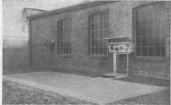
Brückenwaage für Strassenfahrzeuge, Wiegefähigkeit 20 t. Mit Betonbrücke, torsionsfreiem Hebelwerk und verstellbaren Schneiden
