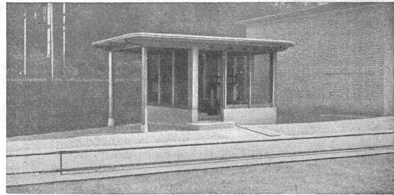
50t Geleisewaage mit armierter Betonbrücke, torsionsfreien Hebeln und verstellbaren Schneiden
