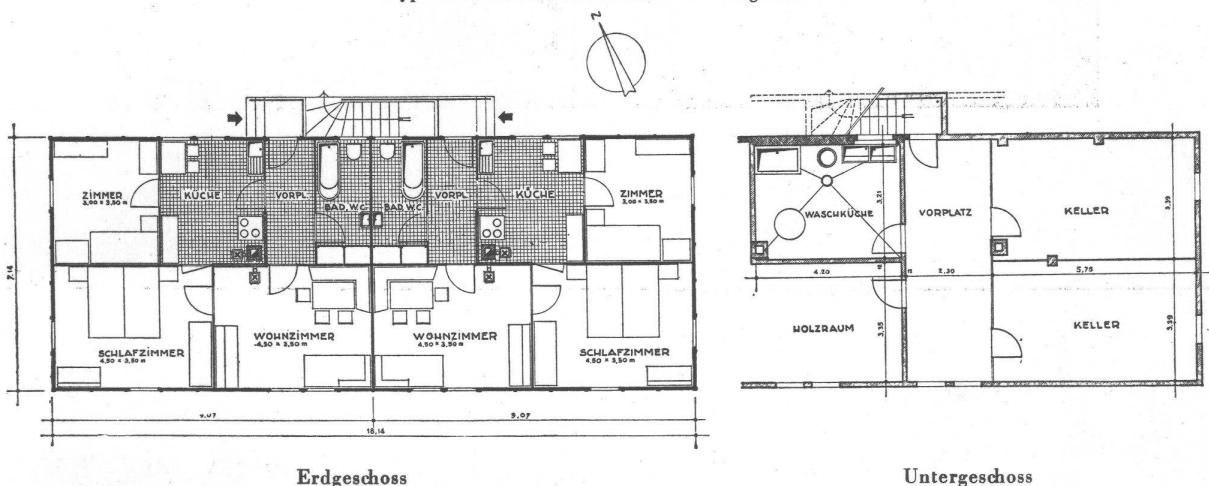
Typ eines Zweifamilienhauses für Angestellte
