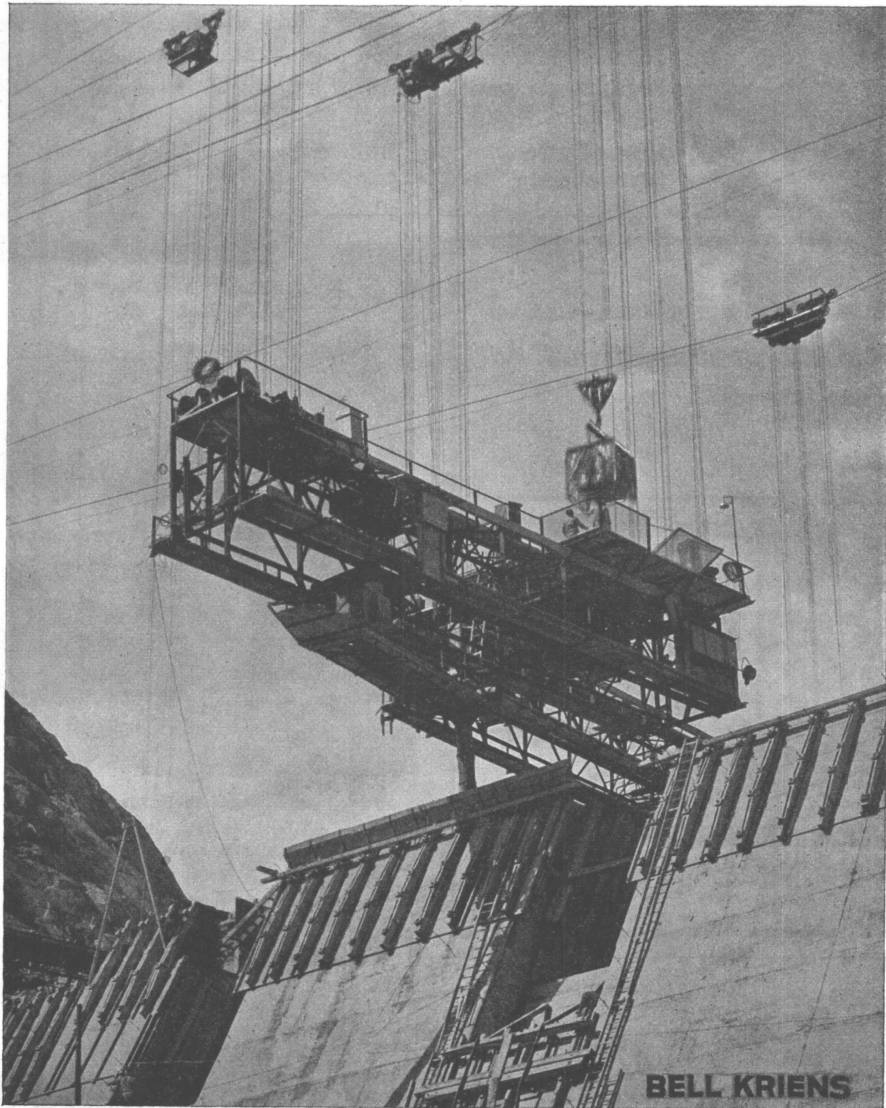
Zwei Bell-Betonierbühnen im Betrieb beim Bau der Staumauer Lucendro
