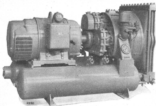
Luftgekühlter Baukompressor 4,5 m³ pro Min.
