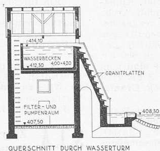
QUERSCHNITT DURCH WASSERTURM
