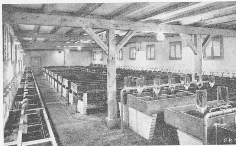
Bild 12. Brutraum
