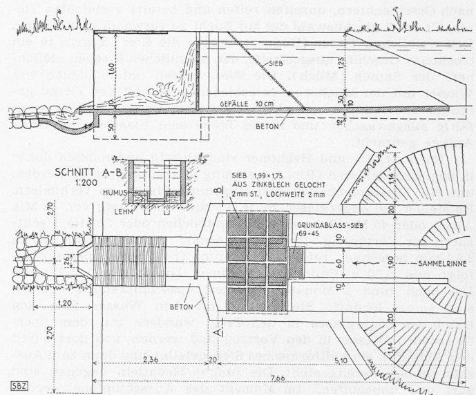
Bild 6. Teich-Auslauf, Einzelheiten 1:100
