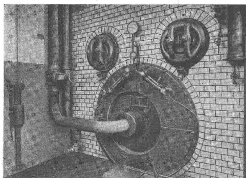
Dampfkessel mit Gasheizung
