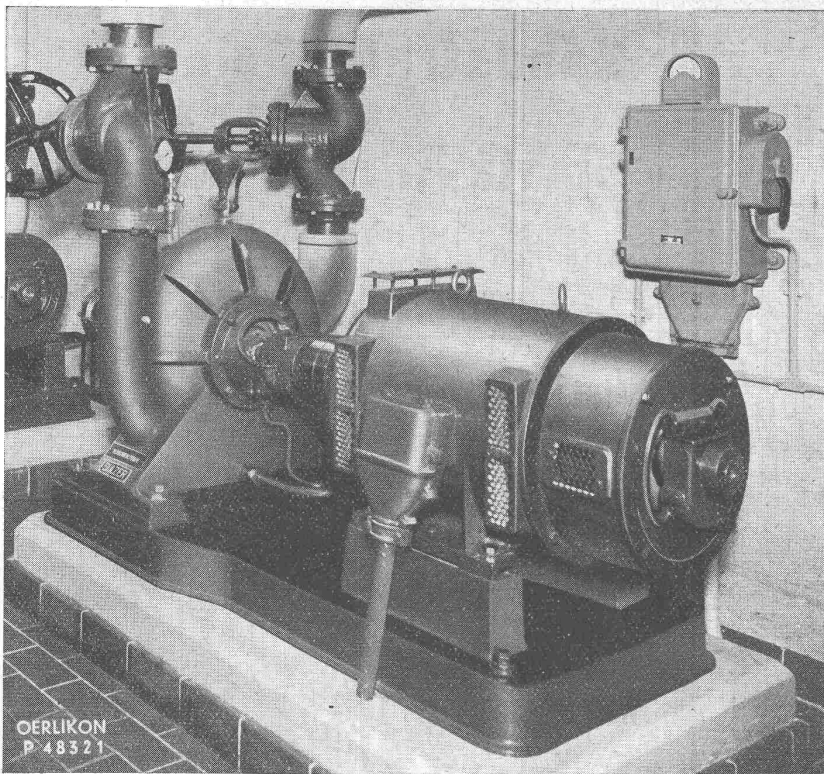
Heisswasserpumpe in der Wärmepumpenanlage E. T. H., angetrieben durch Combi-Motor, 55 PS, 1460 U/min, 380 V, 50 Hz.
