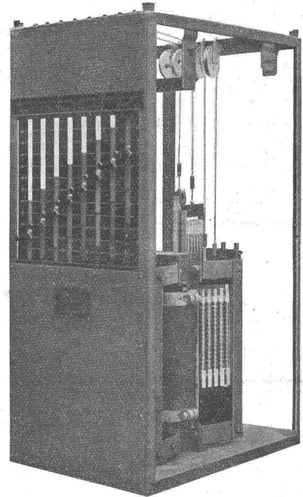
BÜHNEN-LICHTREGLER
