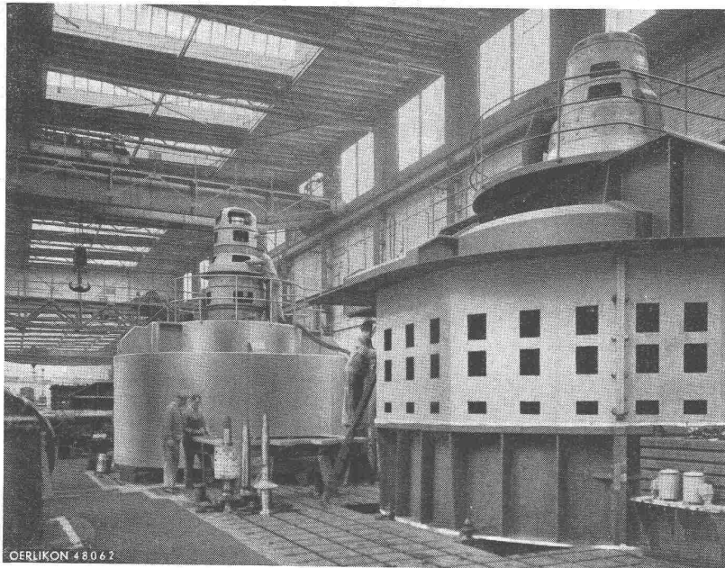
Albula-Generator auf dem Prüfstand in Oerlikon
