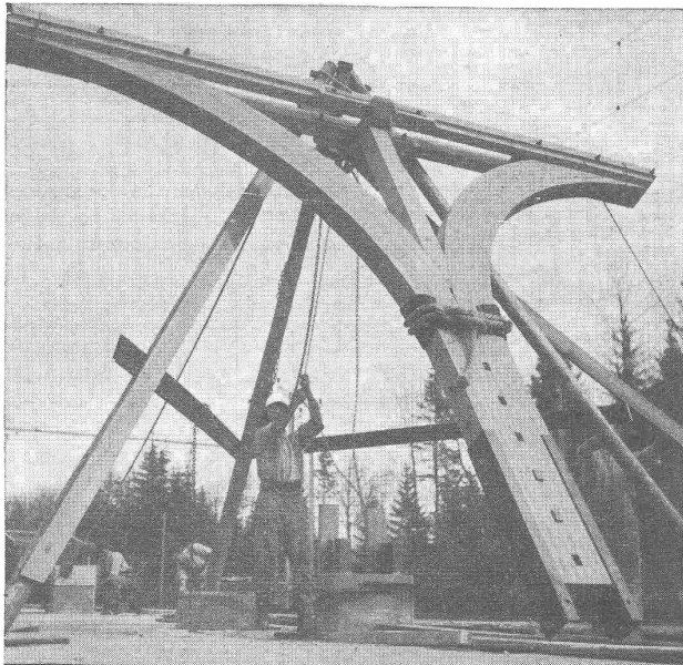
Hetzerträger für Perrondach Bahnhof Ramsei Ersteller: Firma Gribi & Co. A.G., Burgdorf
