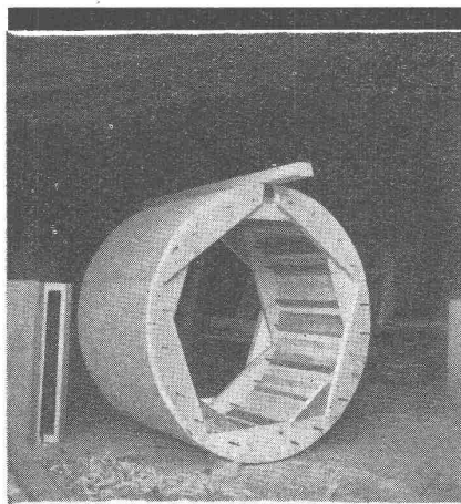
Tunnel- oder Stollenschalung
