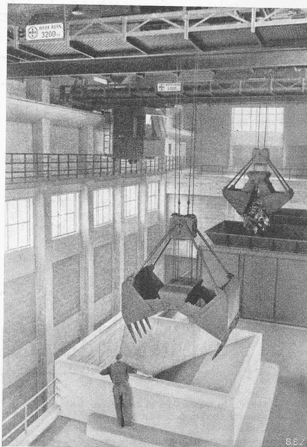
Abb. 5. Greifer-Entleerung in die Fülltrichter 3
