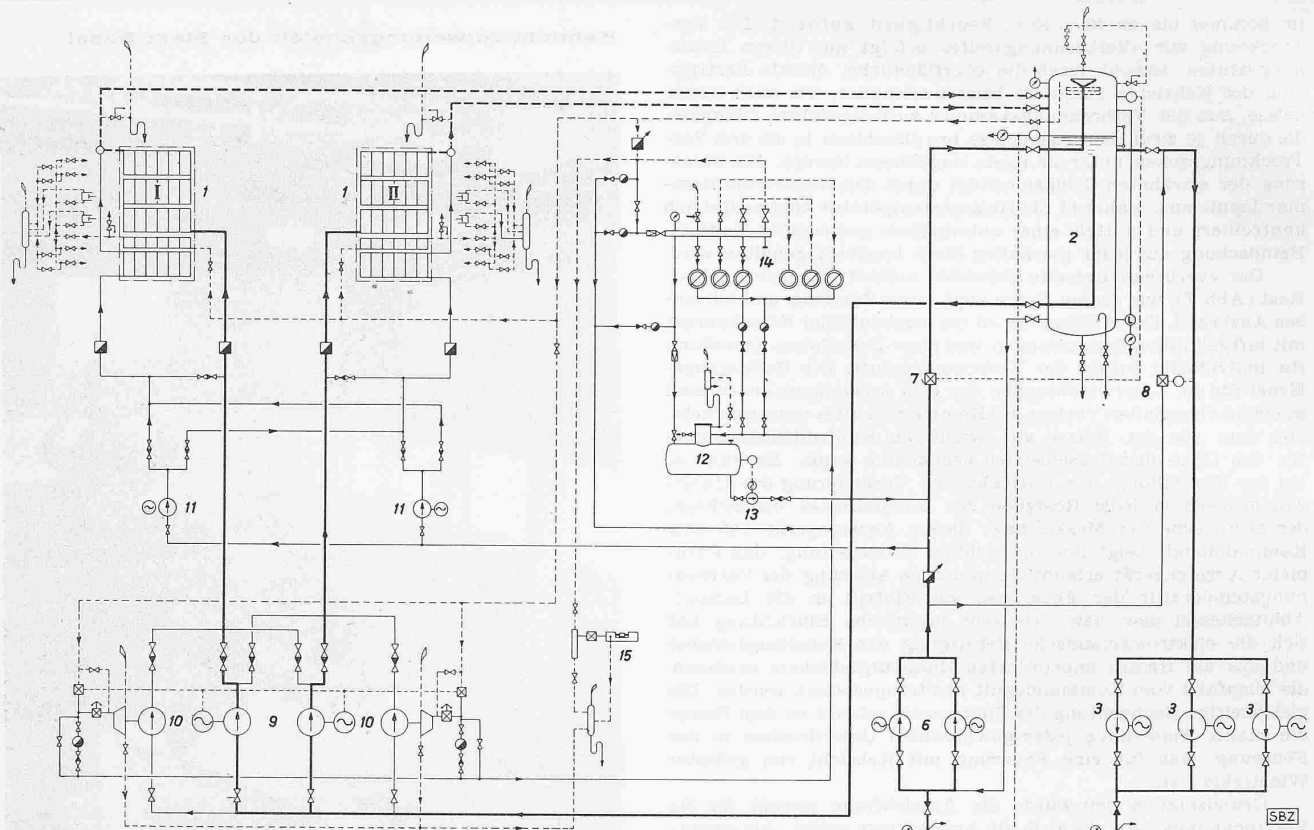
Abb. 10. Leitungsschema in der Zentrale der Kehricht-Verwertungsanstalt Basel
