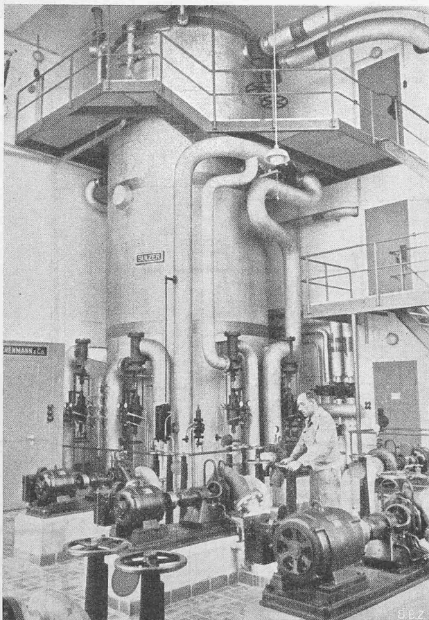
Abb. 9. Wärmезentrale mit Heisswasser-Umwälzpumpen und 98,5 m³-Wärmespeicher
