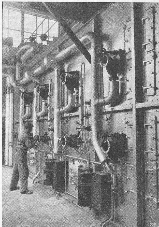
Abb. 8. Bedienung der Lamont-Abhitzeessel (9 in Abb. 3)
