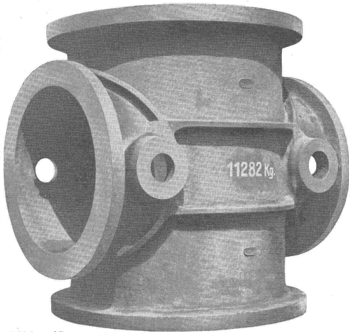
Schiebergehäuse
