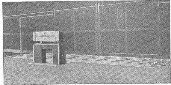
40 t Geleisewaage mit armerter Betonbrücke, torsionsfreien Hebeln und verstellbaren Schneiden.
