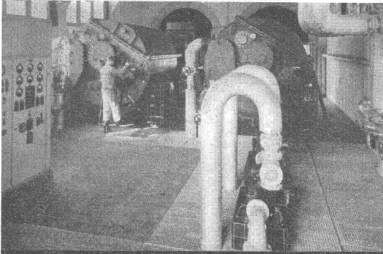
Wärmepumpenanlage der Steckborn Kunstseide A.-G., Steckborn. Zwei Thermoblocs mit einer Heizleistung von je 1,0 bis 1,7 Millionen kcal/h. Jährliche Kohlenersparnis 2 x 2100 Tonnen.
