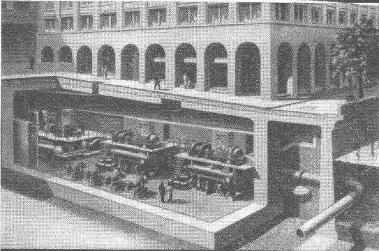
In dieser Wärmepumpenanlage des Fernheizkraftwerkes der ETH Zürich erzeugt jeder der zwei Thermoblocs 1,5 bis 2,5 Millionen kcal/h. Jährliche Kohlenersparnis 2600 Tonnen.
