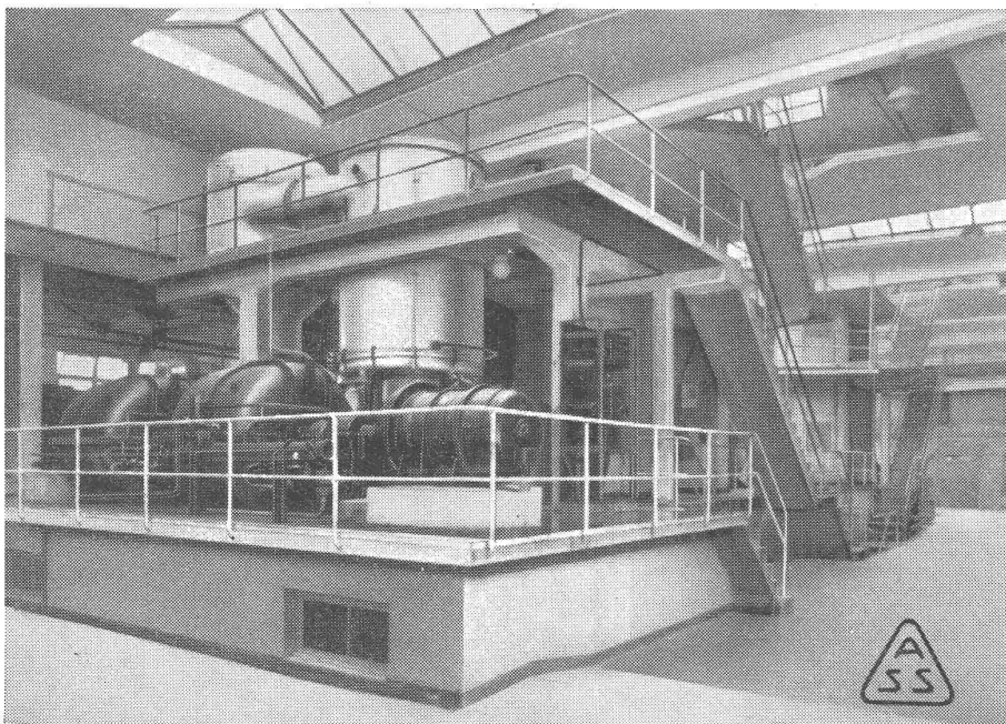
Von uns projektierte u. erstellte Eindampfungsanlage für Milch, Obstsaft etc. mit Wärmepumpe (Turbo-Verdichter)
