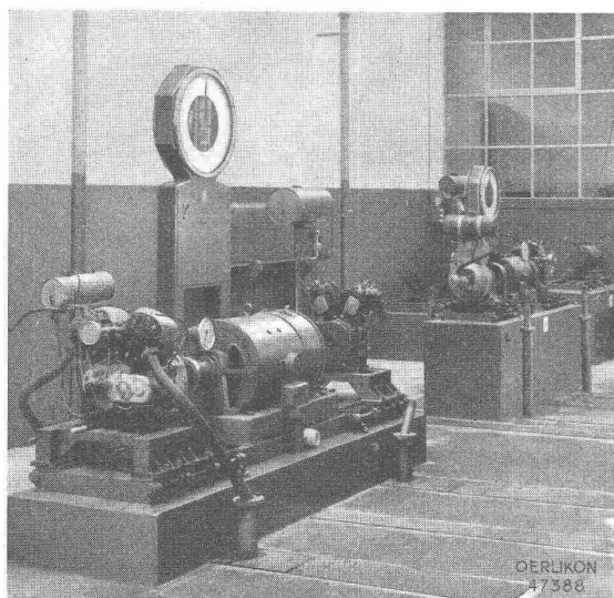
Prüfstände für Kraftmaschinen, ausgerüstet mit Oerlikon-Leistungswaagen
