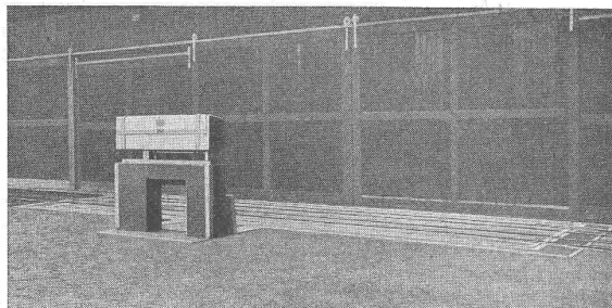
40 t Geleisewaage mit armierter Betonbrücke, torsionsfreien Hebeln und verstellbaren Schneiden.
