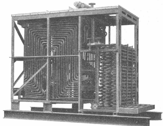
BUSS-La Mont-Heisswassererzeuger für 650 000 WE/h, 205 ° C.
