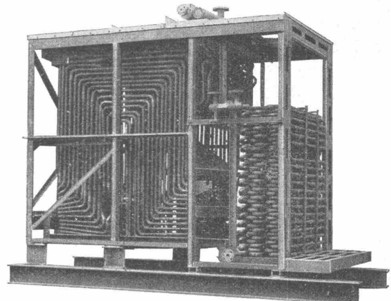
BUSS-La Mont-Heisswassererzeuger für 650 000 WE/h, 205 ° C.
